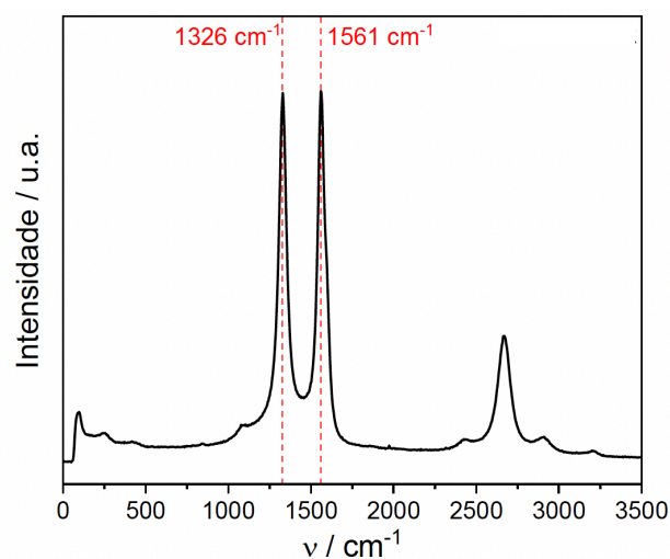
Espectroscopia Raman
