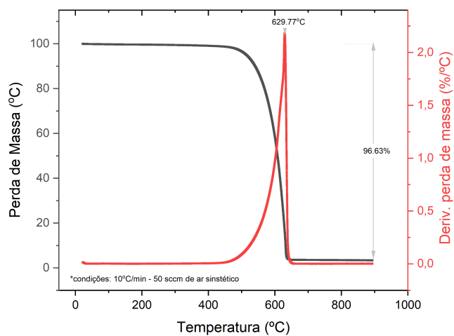
Análise Termogravimétrica
